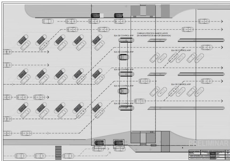
Imagen 07- Plan Maestro de la Propuesta de Re funcionalización del Centro de Frontera. Sector Ingreso al país-casillas de control migratorio / aduanero / requisa vehículos
