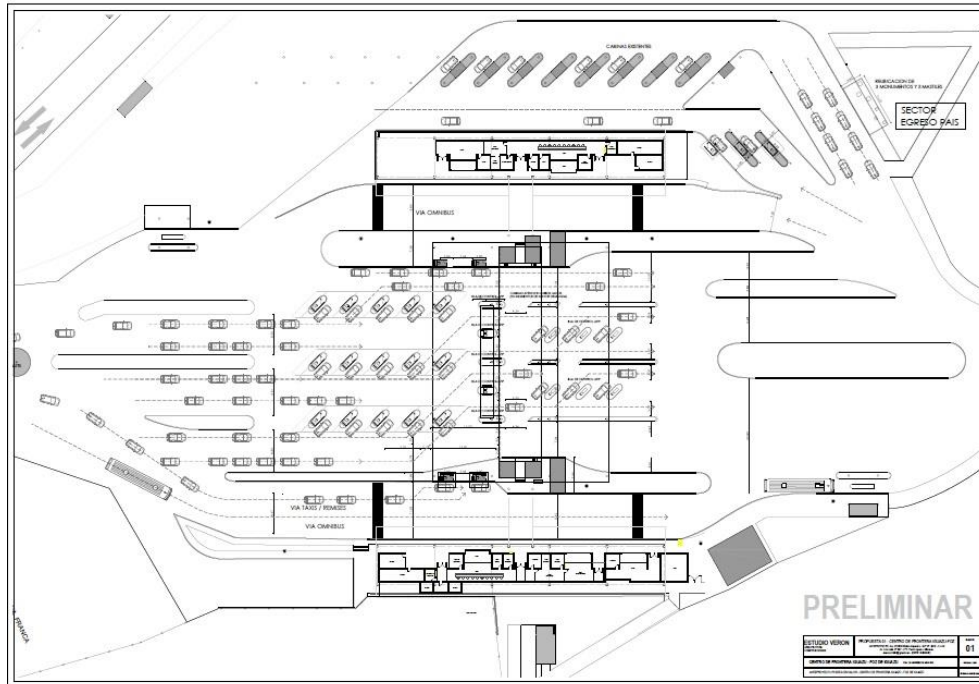
Imagen 06- Plan Maestro de la Propuesta de Re funcionalización del Centro de Frontera.
