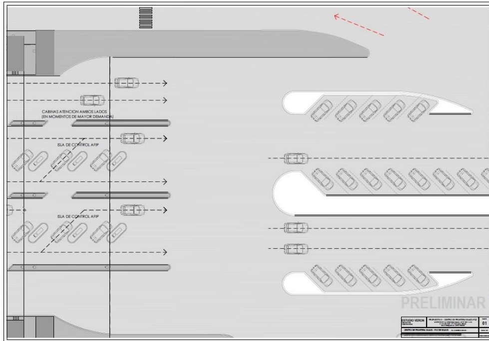
Imagen 08- Plan Maestro de la Propuesta de Re funcionalización del Centro de Frontera. Sector Ingreso al país-casillas de control aduanero / requisa vehículos-estacionamiento
