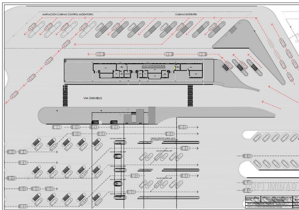
Imagen 09- Plan Maestro de la Propuesta de Re funcionalización del Centro de Frontera. Sector Egreso -casillas de control migratorio
